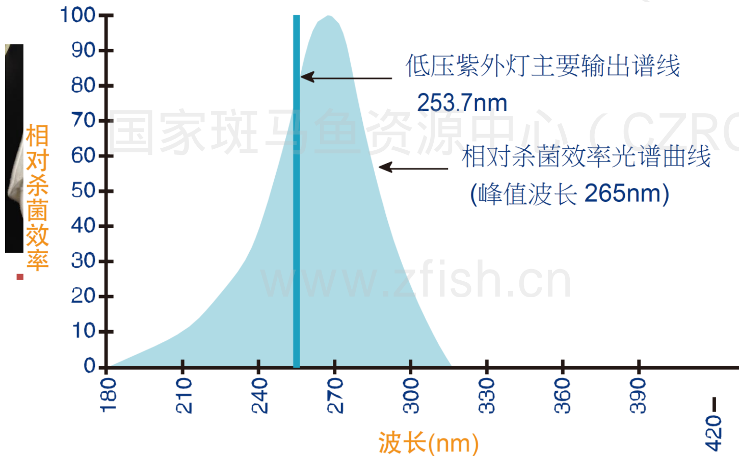
低压紫外灯杀菌效率图示
